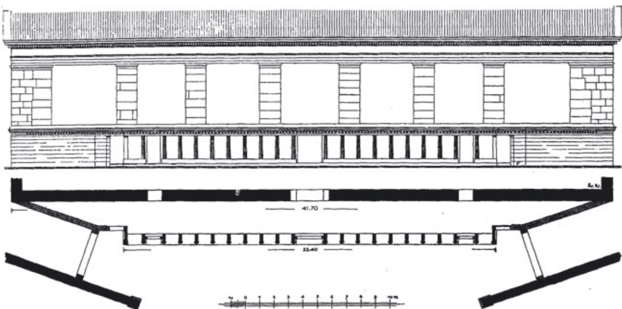
Abb. 753: Bühnengebäude, Rekonstruktion der ›Thyromata-Wand‹ (Phase 2) (nach HEBERDEY u. a. 1912)
