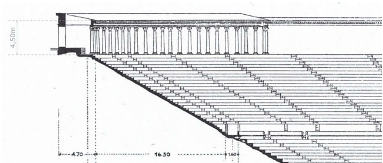
Abb. 828: Querschnitt durch das Theater mit Rekonstruktion der Portikus (HEBERDEY u. a. 1912, Maßangabe ergänzt)
