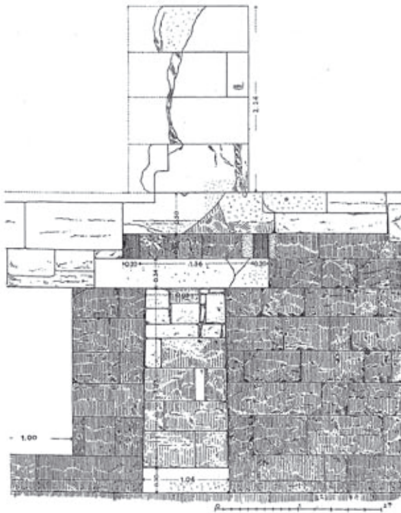
Abb. 751: Bühnengebäude, Situation Tür c (Phase 1) u. ›Thyromata-Wand‹ (Phase 2) (nach HEBERDEY u. a. 1912)
