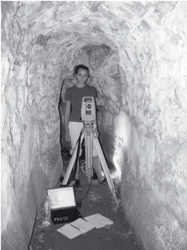
Abb. 826: Aristion-Leitung während der Bauaufnahme. Im Streckenabschnitt II hat die Wasserleitung Durchgangshöhe
