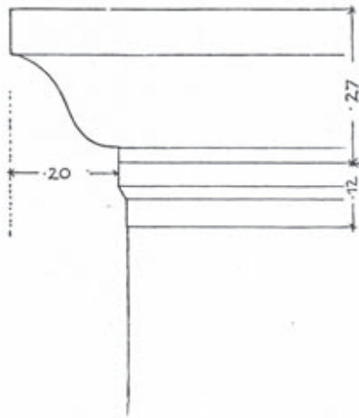
Abb. 790: Orchestra, Wand X: Oberprofil a) nach HEBERDEY u. a. 1912; b) aktuelle Befundsituation
