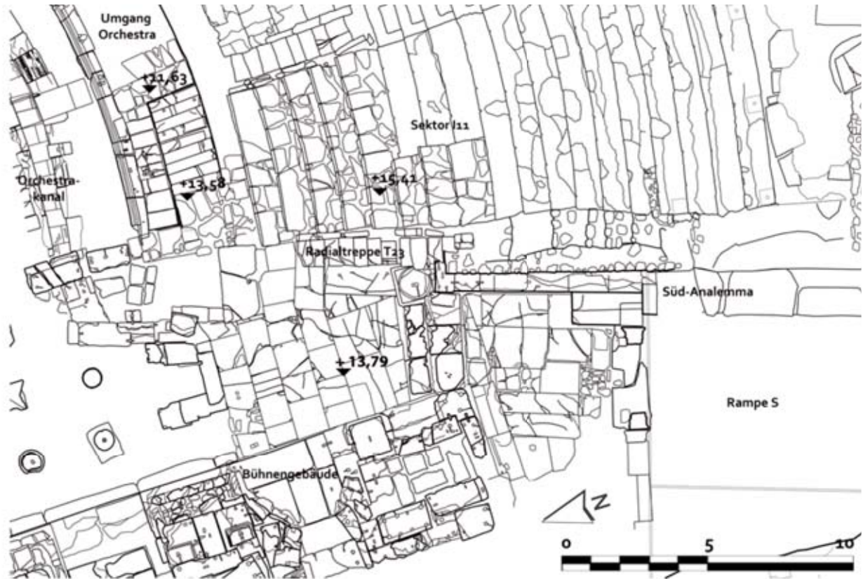
Abb. 788: Plattform am Beginn des (versetzten) südl. Analemma oberhalb der Süd-Parodos: Aufsicht
