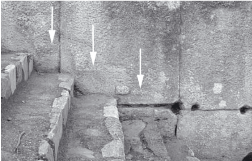
Abb. 816: Südl. vomitorium ES1, Treppenaufgang. Wandansicht mit Kontaktstellen für die ehemaligen Stufenquader
