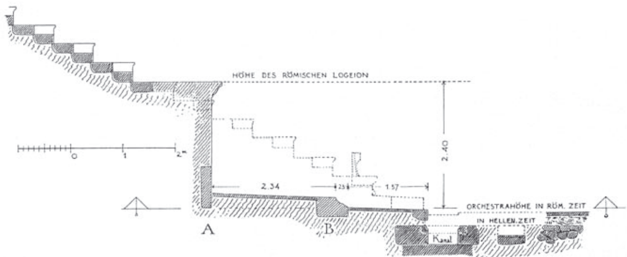
Abb. 760: Koilon, Rekonstruktion der unteren – später entfernten – Sitzreihen (nach HEBERDEY u. a. 1912)
