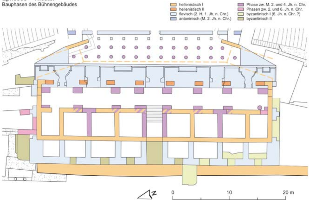
Abb. 758: Bühnengebäude, Übersicht Bauphasen
