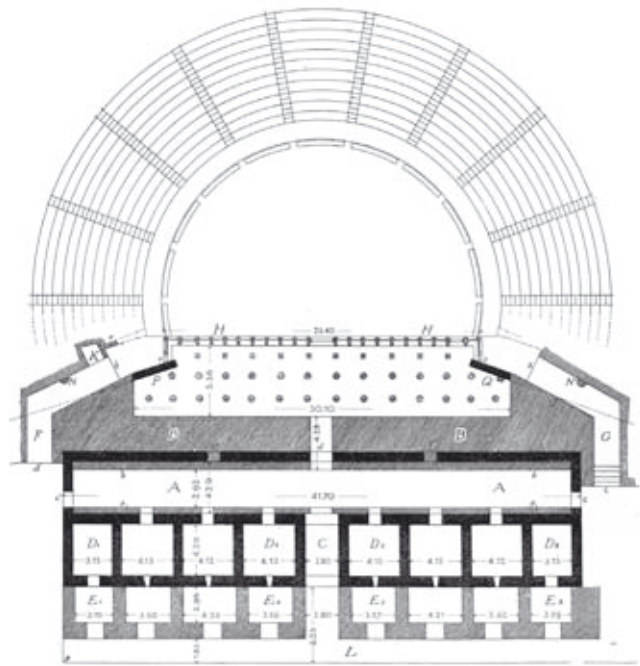
Abb. 784: Bühne u. Orchestra nach Errichtung der scaenae frons (nach HEBERDEY u. a. 1912)
