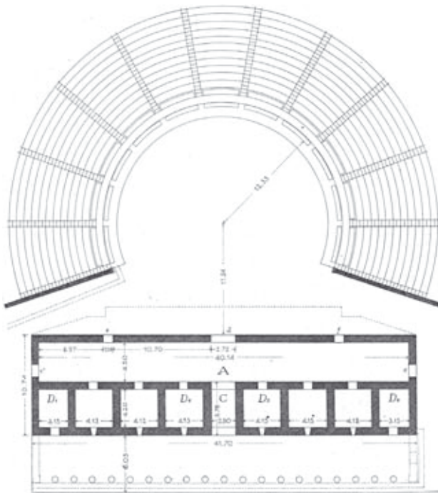
Abb. 783: Bühne u. Orchestra in hellenistischer Zeit (nach HEBERDEY u. a. 1912)
