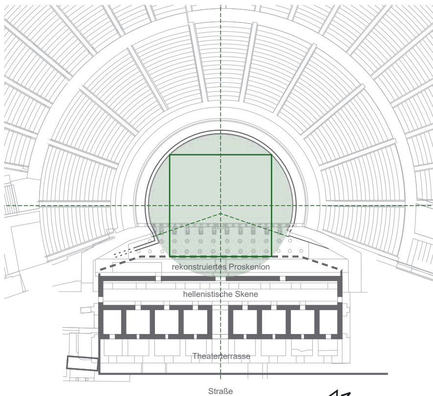
Ephesos - Theater Konstruktionsschema nach Vitruv
