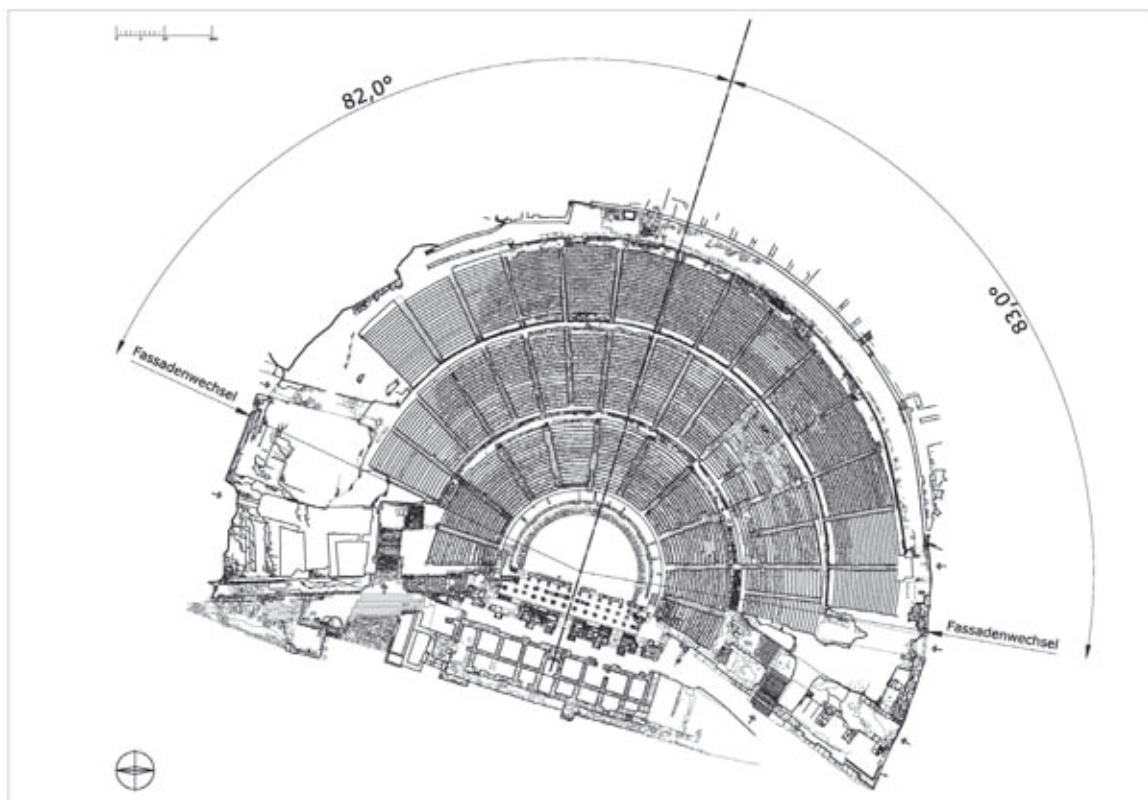
Abb. 765: Nördl. u. südl. Außenwand des Theaters, Position des Fassadenwechsels
