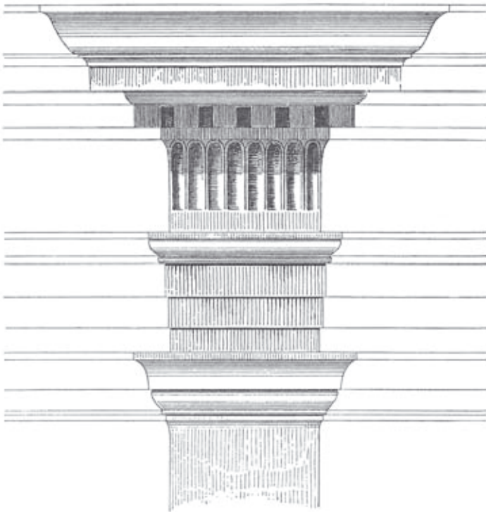
Abb. 817: Süd-Analemma. Oberer Abschluss der Pilaster, Rekonstruktion (HEBERDEY u. a. 1912)
