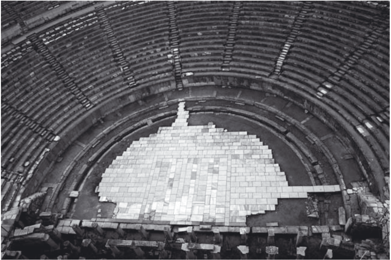
Abb. 762: Gesamtansicht Orchestra, hell. Ringkanal mit regelmäßig angeordneten Trittsteinen
